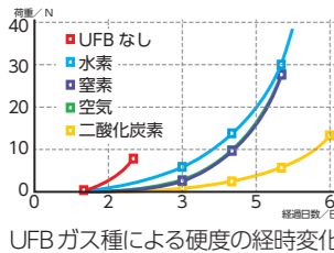
UFBガス種による硬度の経時変化
